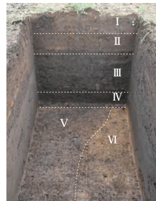
写真4 基本層序 (16トレンチ南壁)
