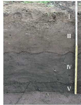
写真3 基本層序 (9トレンチ東部南壁)
